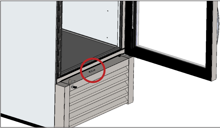
Rys. 1. Wykręcić górną śrubę z kratki żaluzyjowej.
