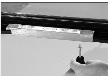
Abb. 2. Transportbügel der Glasschwingtür entfernen, falls vorhanden. Nicht wegwerfen
