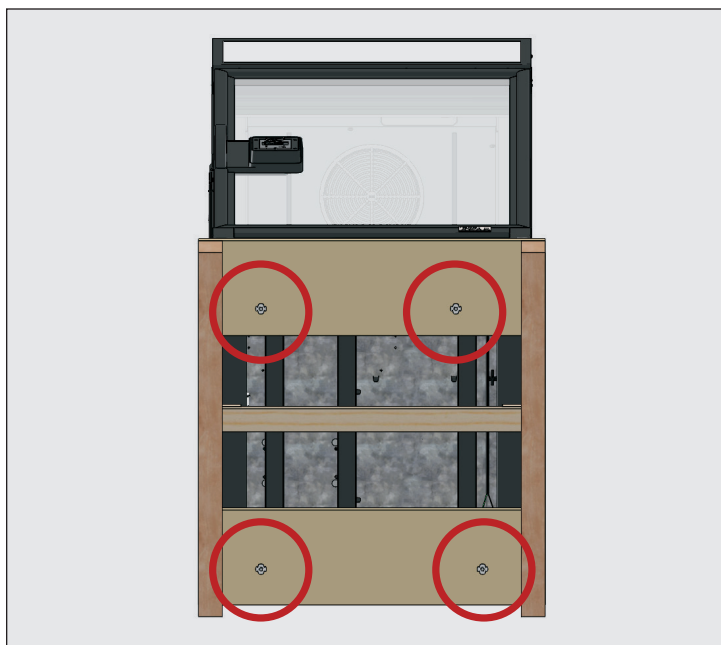
Рис. 3. Расположение транспортных болтов.
