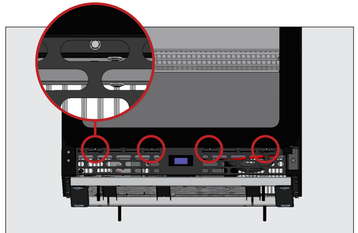
Fig. 3. Retire los pernos de la rejilla frontal para tener acceso a los pernos de transporte.
