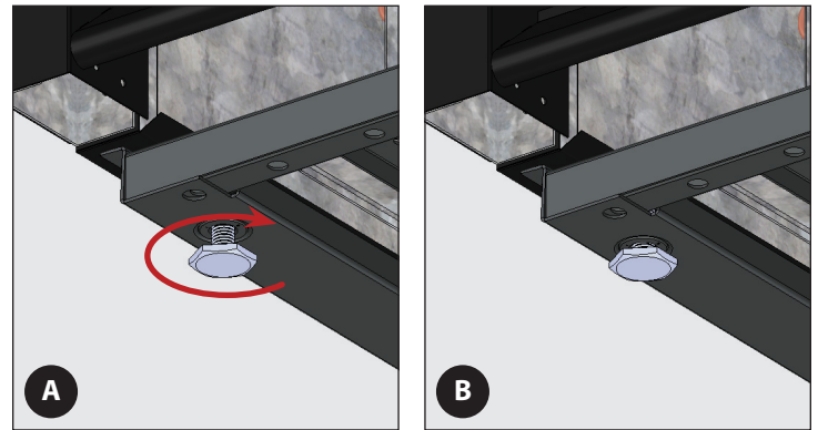
Fig. 2. Gire los tornillos de nivelación en sentido horario para bajar la unidad.
