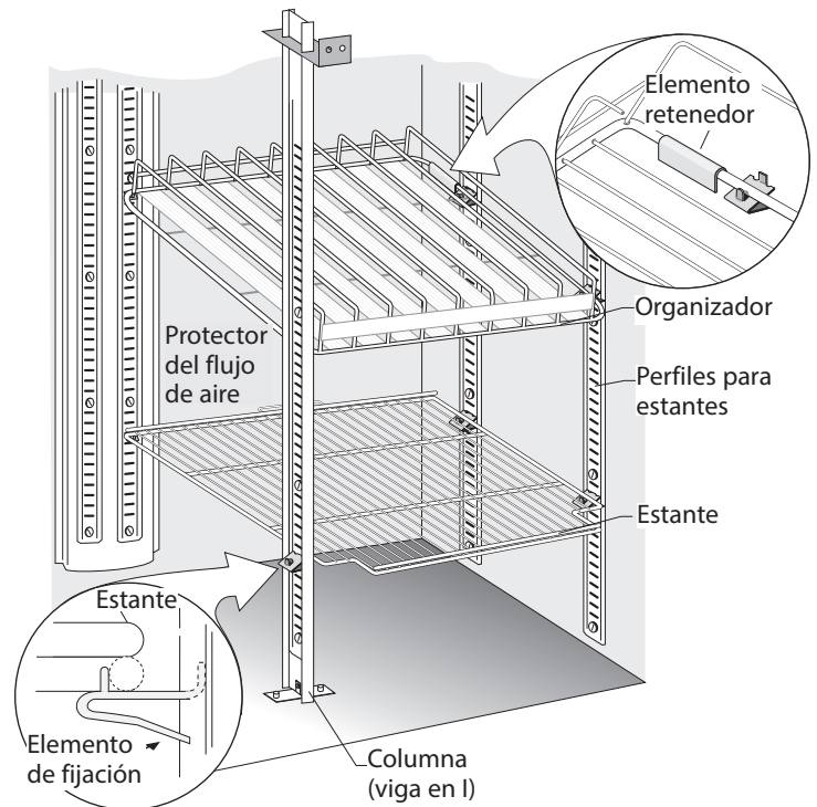
Fig. 5. Elemento de fijación instalado.
