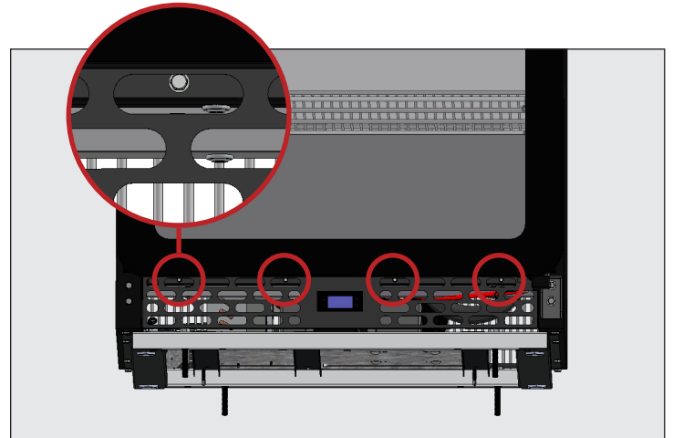
Fig. 3. Retirez les boulons de la grille avant pour accéder aux boulons de transport.
