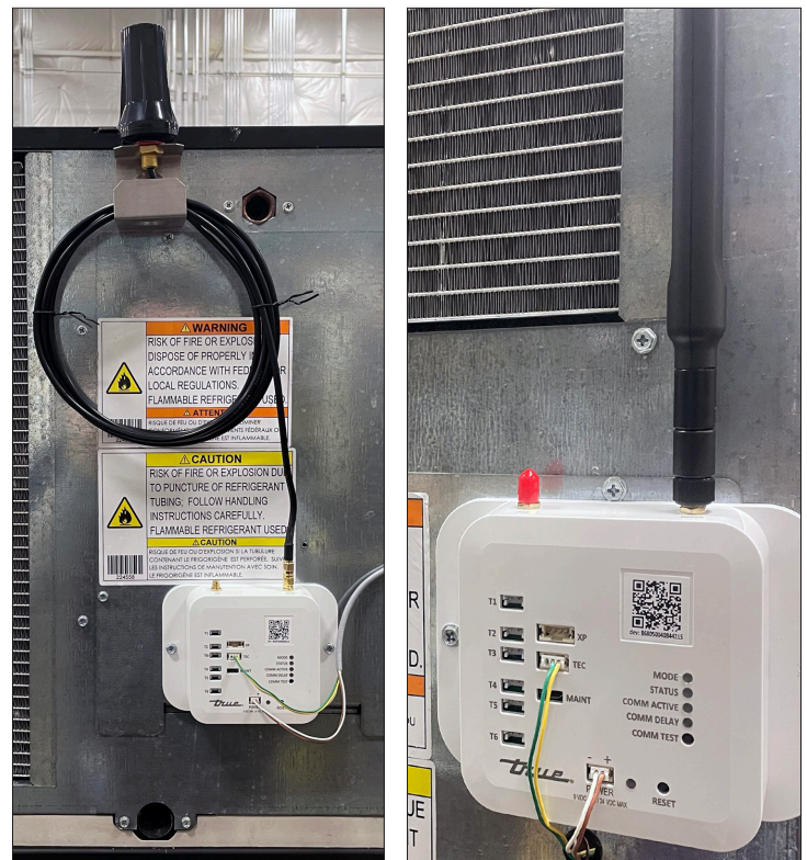
Рис. 3. Антенна на модеме. Ваша антенна может отличаться.
