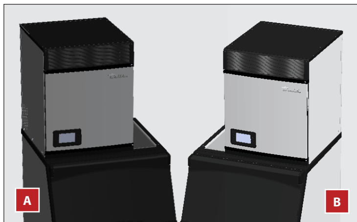
Рис. 3. 22-дюймовый льдогенератор, установленный слева (А) и справа (В) на 30-дюймовом контейнере с помощью переходного устройства.
